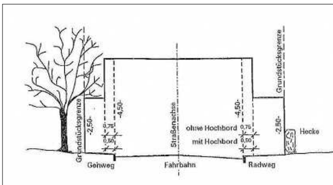
Lichtraumprofil
