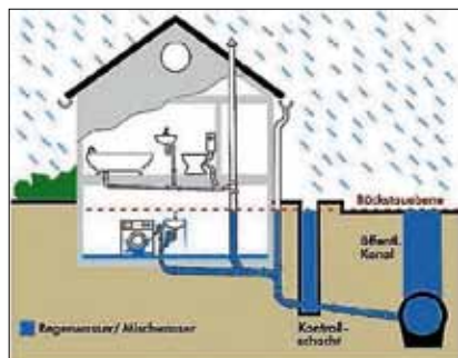
Bild 1: Rückstauenebene (Quelle: DWA) Foto: Quelle: DWA
