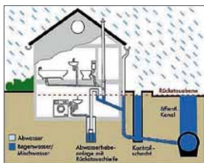
Bild 2: Abwasserhebeanlage (Quelle: DWA) Foto: Quelle: DWA
